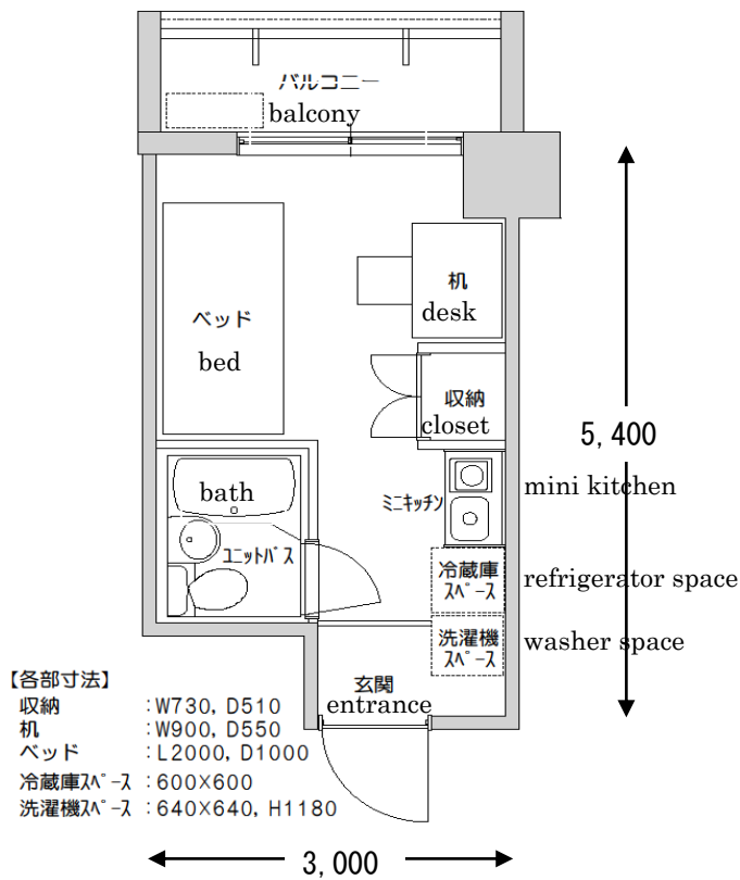
《A棟居室平面図—Building A》
